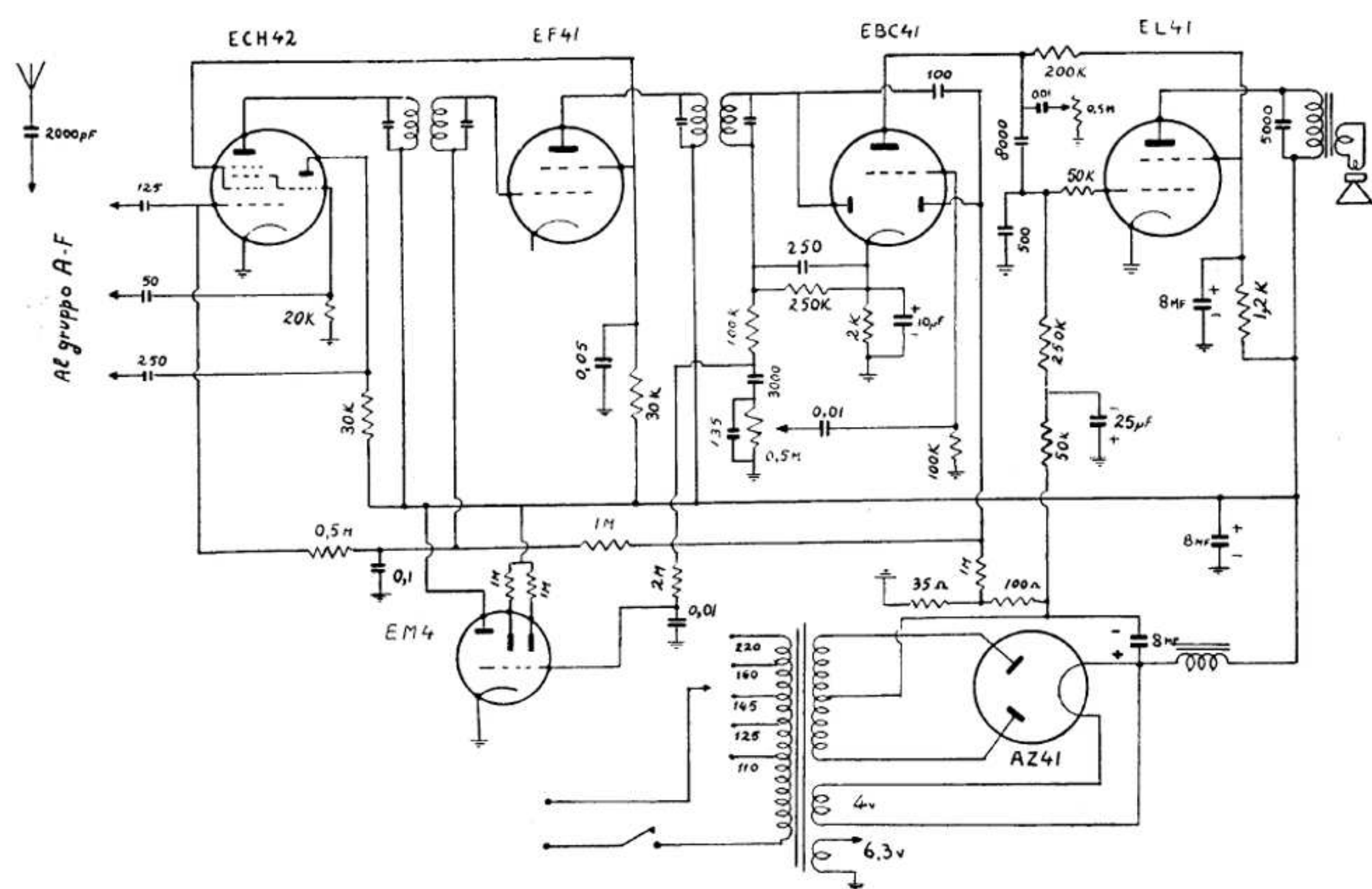
AITAR - Mod. MR15 E. Lunghezza d'onda in metri: 13-27; 27-55; 55-170; 180-580. Media frequenza 467 kc/s. Tensione 1° elettrolitico 315 volt, al 2° elettrolitico 257. Potenza d'uscita 4,5 watt.
